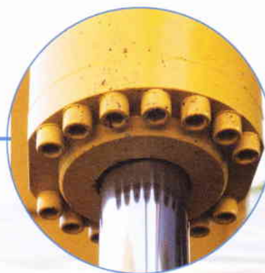
CILINDRO ALZATA PRIMO BRACCIO Ø INTERNO 125 mm
